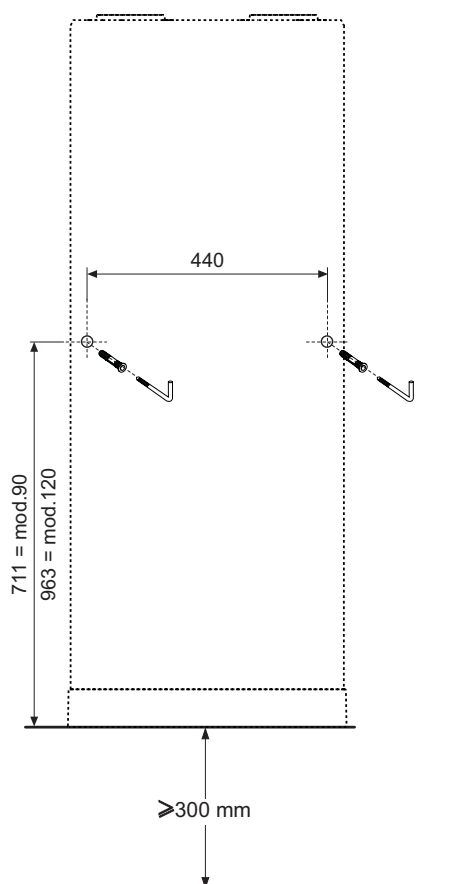
fig. 50 - Indicazione foratura
