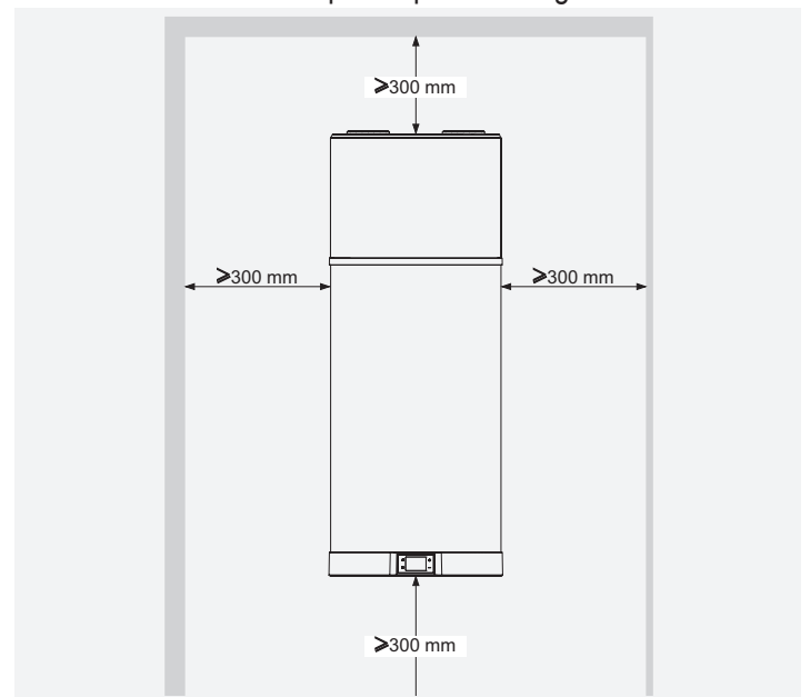
fig. 49 - Spazi minimi
